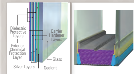
12 Layer Glass
