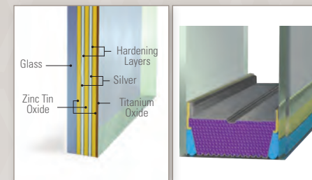
8 Layer Glass
