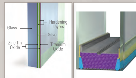
6 Layer Glass
